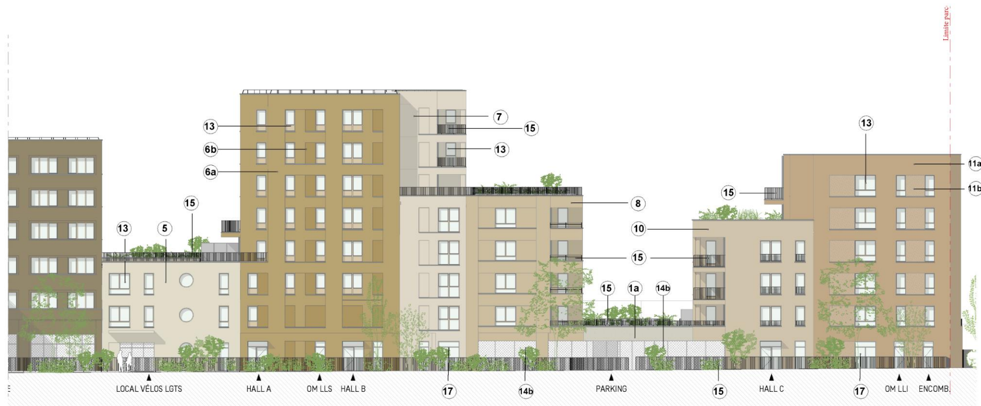
FACADE NORD _ VOIE NOUVELLE VULCAIN
