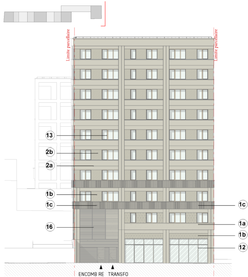
FACADE EST _ AVENUE JEAN JAURES
